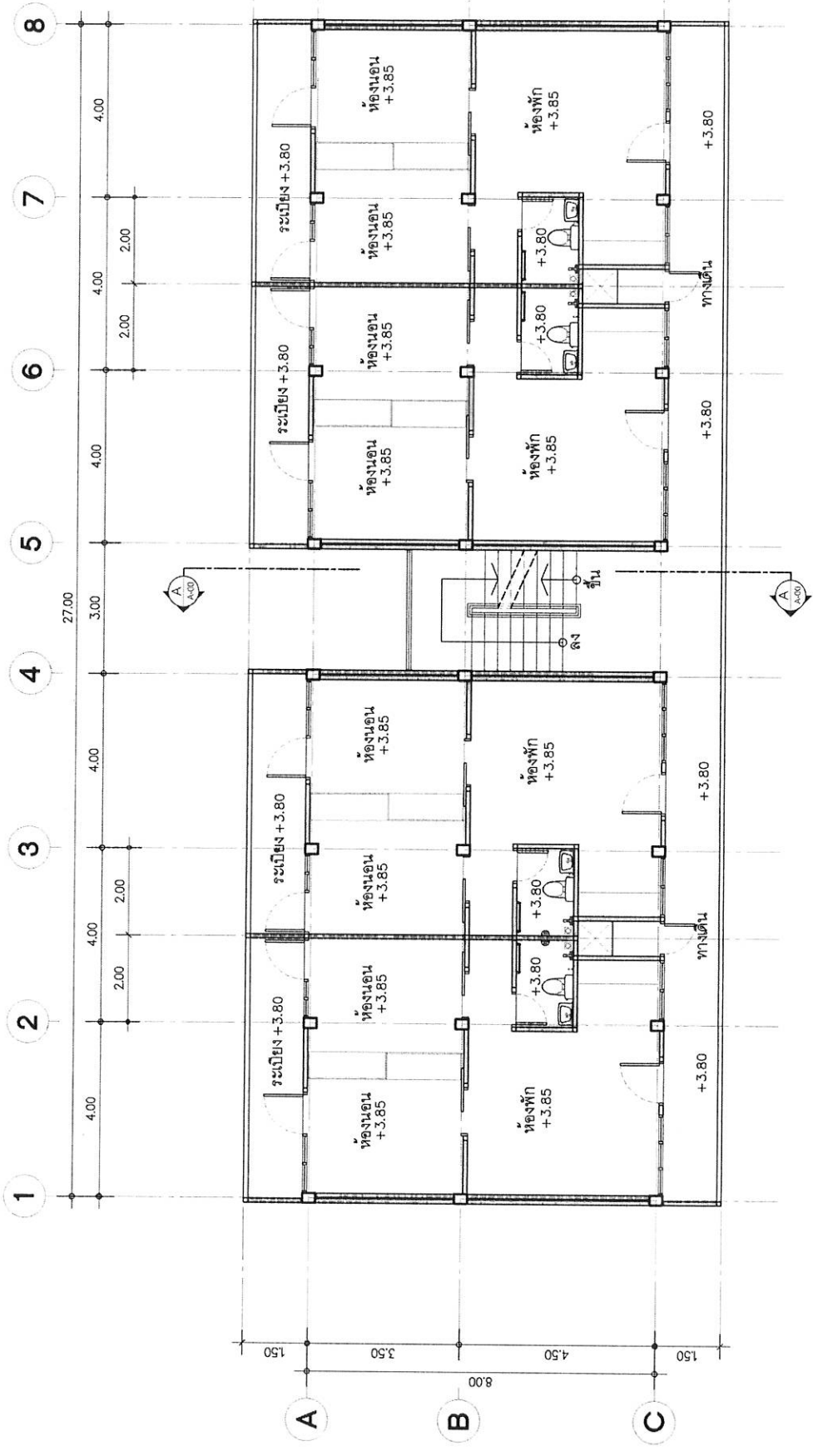
3 4 2 1 แผนผังพื้นที่ 2-3 (ก่อนการปรับปรุง) SCALE 1:100
